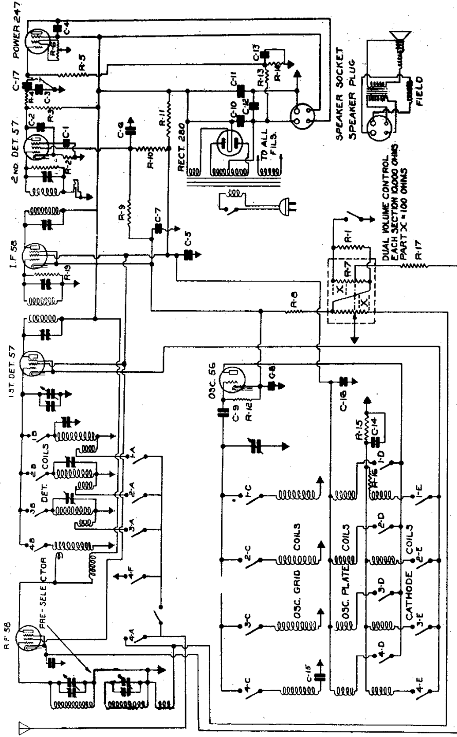
SCHMATIC DIAGRAM DRAGON MODEL 10 SUPER HET
