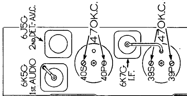
Fig. 6—I. F. Compensators
